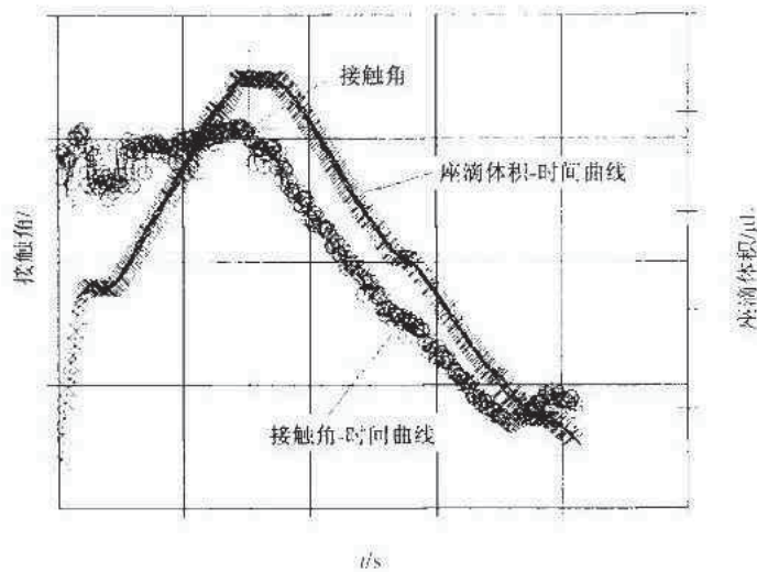
图3 前进接触角随时间的变化示意图
