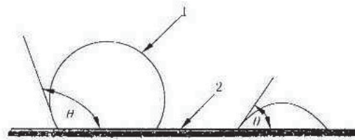
图 1 接触角示意图
